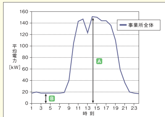
最大ピーク電力を記録した日の電力の変化 (2)
