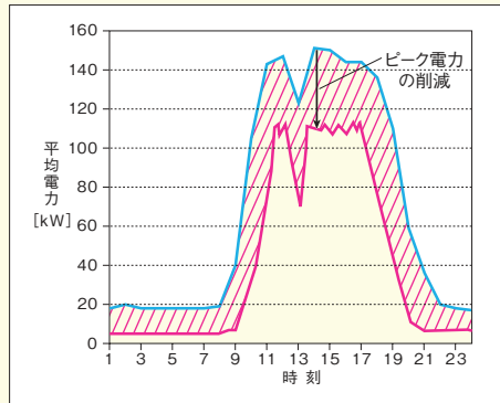
事業所全体の電力変化
