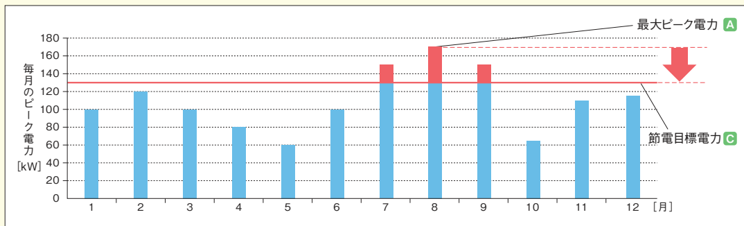
毎月のピーク電力変化
