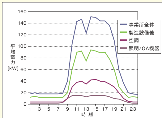
最大ピーク電力を記録した日の電力の変化 (1)
